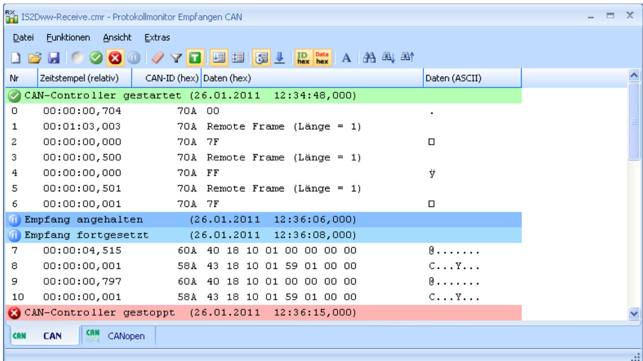
Abbildung 21: Protokollmonitor Empfangen CAN - Modus: Scrollen
