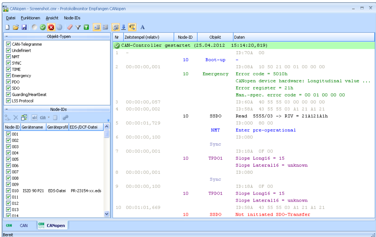
Abbildung 23: Protokollmonitor Empfangen CANopen
