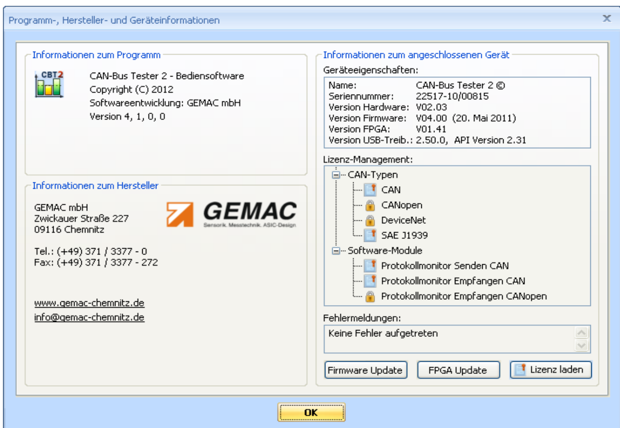
Abbildung 26: Lizenz Management im Informationsdialog
