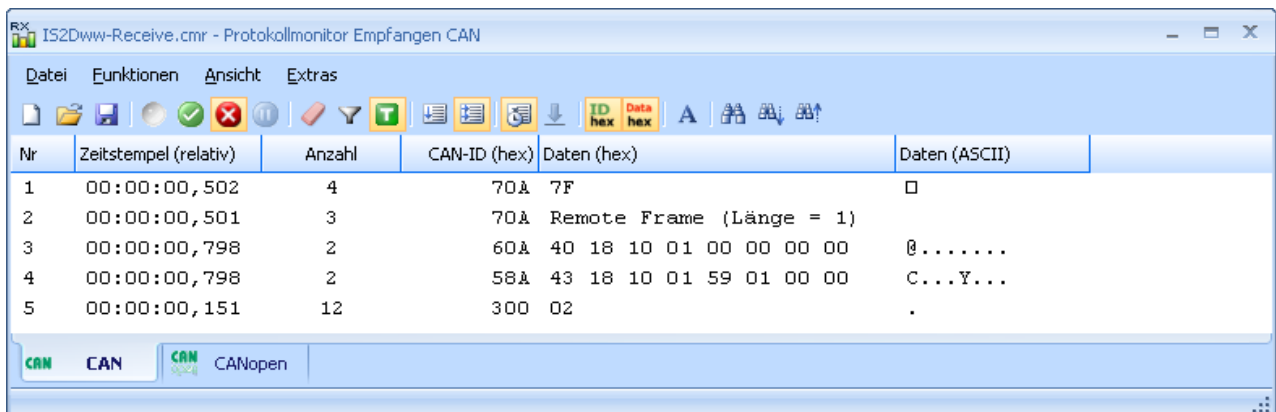
Abbildung 22: Protokollmonitor Empfangen CAN - Modus: Überschreiben
